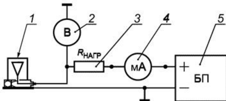
Рисунок 1 - Обобщенная схема для определения начального рабочего напряжения (тока) вибропреобразователей с выходом по напряжению (току)
